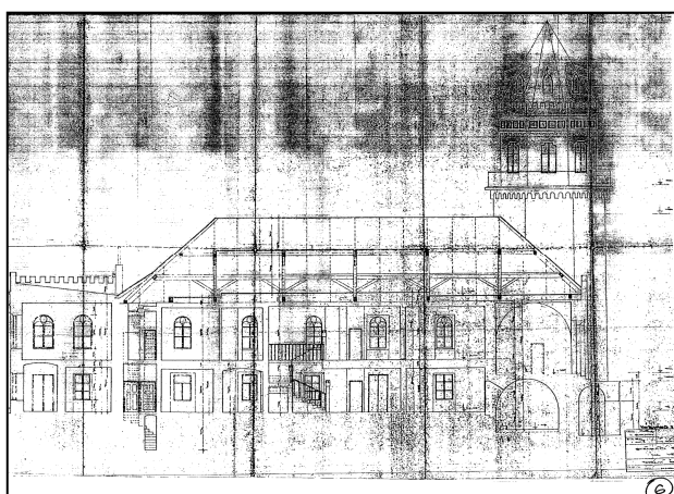
Obr. 6: Veselí, zámek, výkres z roku 1976, podélný řez, autor Střední průmyslová škola stavební v Plzni (Atelier Soukup OPL Švehla s.r.o.).
