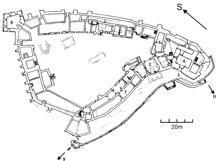
Vlevo hrad Sümeg na plánu G. Turca z roku 1569. Vpravo současná podoba hradu Sümeg. Popsány jen starší stavby: 1 – první brána, 2 – druhá brána, 3 – parkán, 4 – věž, 5 – kaple, 6 – třetí brána, 7 – palác, 8 – bastion, 9, 10 – napojení hradeb městečka.
