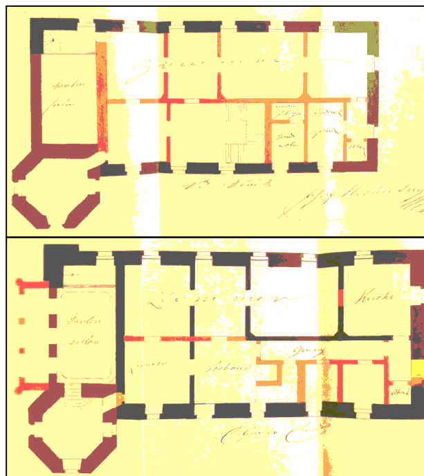
Obr. 4: Veselí, výřez z plánu přestavby zámku, nahoře půdorys přízemí, dole půdorys patra (citace v pozn. 1).
