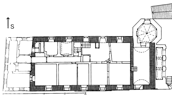
Obr. 7: Veselí, zámek, plán přízemí, autor J. Úlovec. Křížky označil autor dochované zdivo pravděpodobně z 16. století, mladší zdivo převážně z období po 1863 neoznačeno. (druhá citace v pozn. 3).
