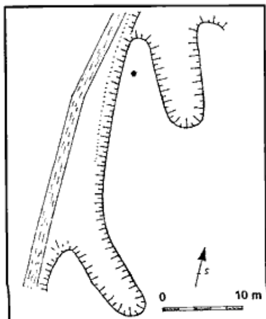
Hrádek (Čebříkov) - plánek autora z doby okolo r. 1985
