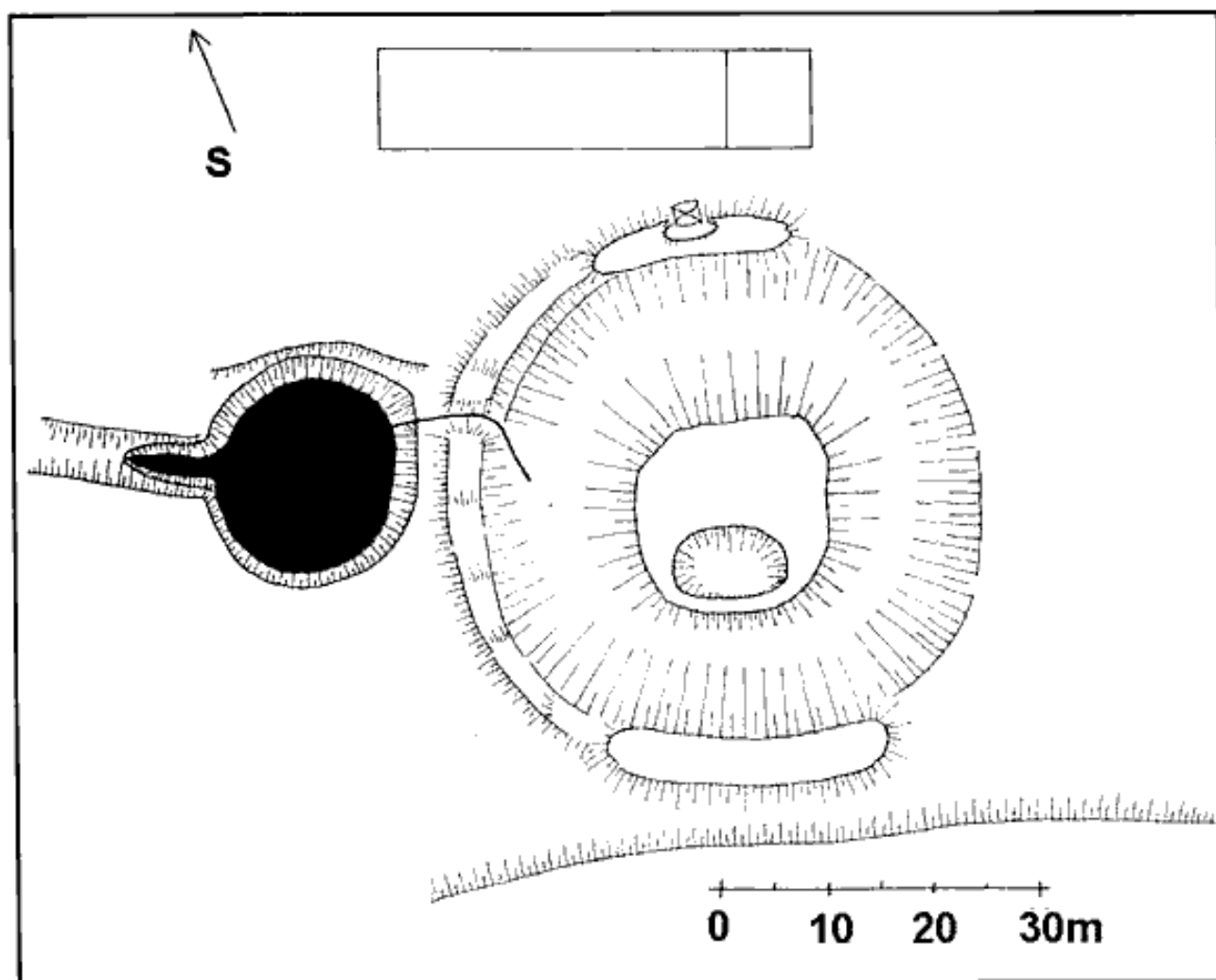
Obr. 3: Černýš (Benešov), plán tvrziště, odvozený ze zaměření z roku 1995. Kresba autor
