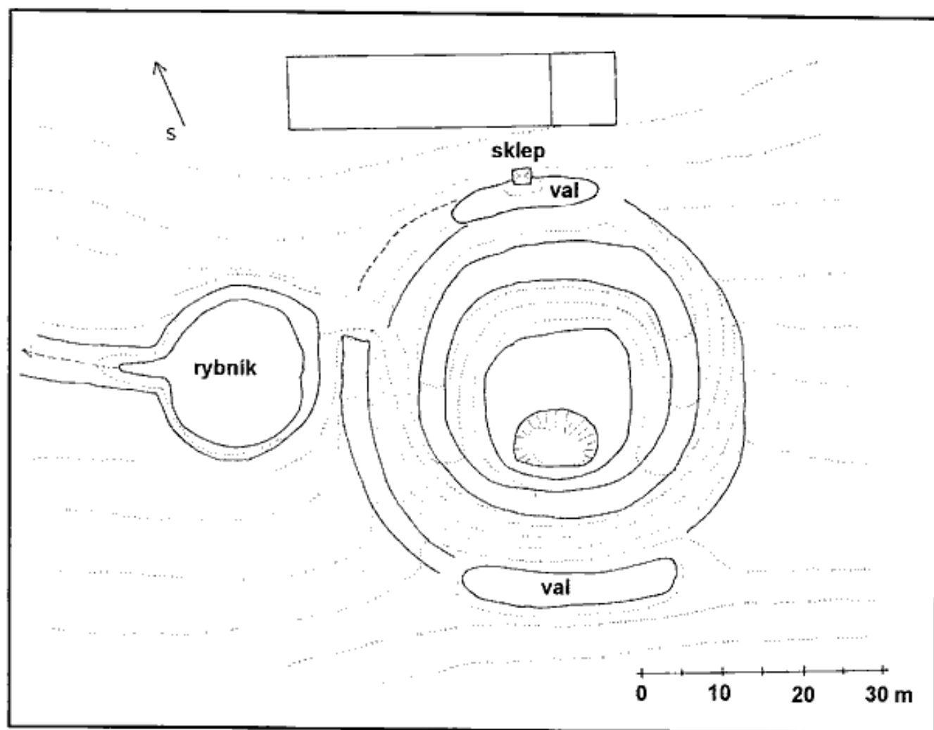
Obr. 2: Černýš (Benešov), celková situace tvrzště. Zaměřili K. Tomíček, T. Tomíček a J. Úlovec roku 1995, vynesl T. Tomíček, kresba autor
