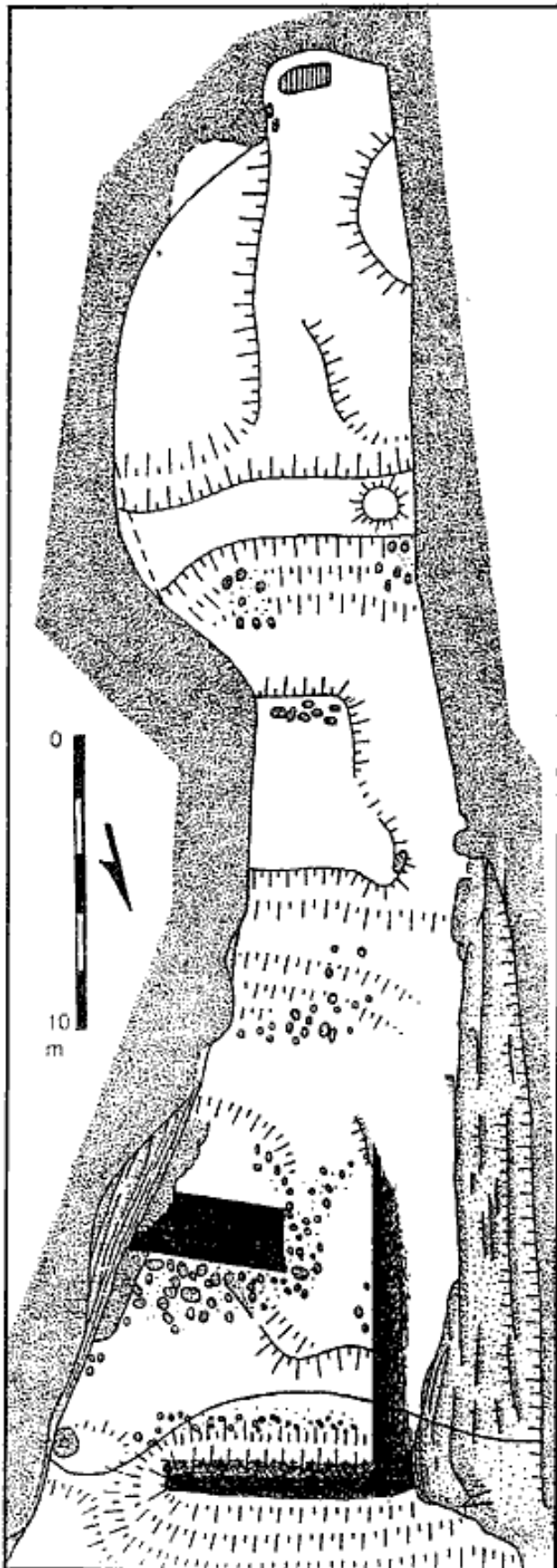
Rytířská jeskyně. Zdivo východ - západ středověké, zdivo sever - jih novodobě z počátku 20. století (měřeno pásmem na jaře 1995, zaměření a kresba autor)
