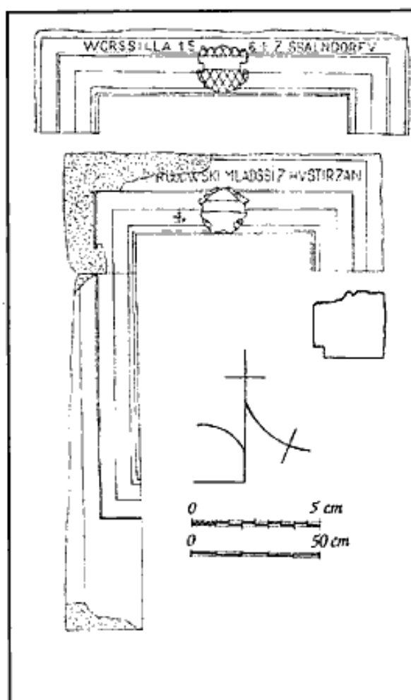
2 - Ostění z libotovské tvrze, dole kamenická značka a profil ostění. Zaměření J. Slavík.
