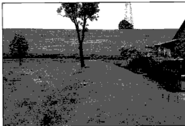
Obr. 8: Lhota (okr. Třebíč), další z hrází kaskády rybníků s bočním bezpečnostním přelivem od jihozápadu (foto L. Krčmář)
