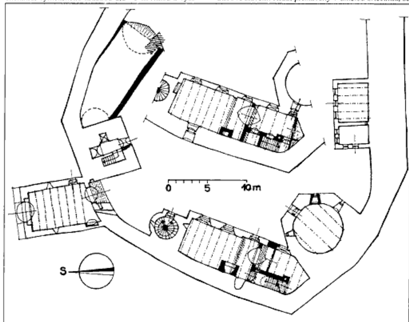
Nový hrad. Náčrt půdorysu přízemí a severovýchodního suterénu hradu - stav v. 2002. Nahoře první patro západní budovy. Černé zdivo z l. 1990 - 2002, šrafování v průběhu přestavby zhořelé. Kresby autor, 2002
