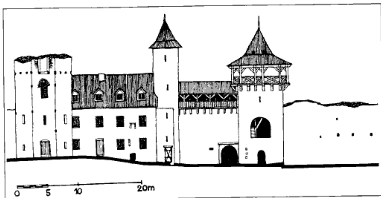
Nový hrad. Rozvinutý pohled na dvorní fasády hradu. Stav r. 2002
