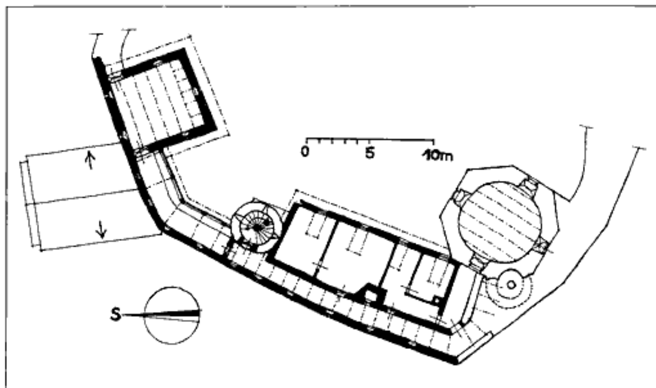
Nový hrad. Náčrt půdorysu druhého patra hradu, stav r. 2002. Černé zdivo z l. 1990 - 2002, šrafované v průběhu přestavby zbořeně
