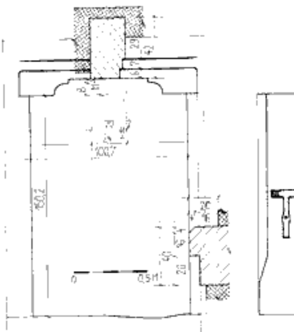
Mladotice, čp. 11, sedlový portál od severu (ze sklepa, zadní strana) a jeho pravá stojka (od jihu, z prostoru pod verandou, přední strana). Šrafování vlastní portál, křížkování okolní zdivo a strop. Zaměření autoři.
