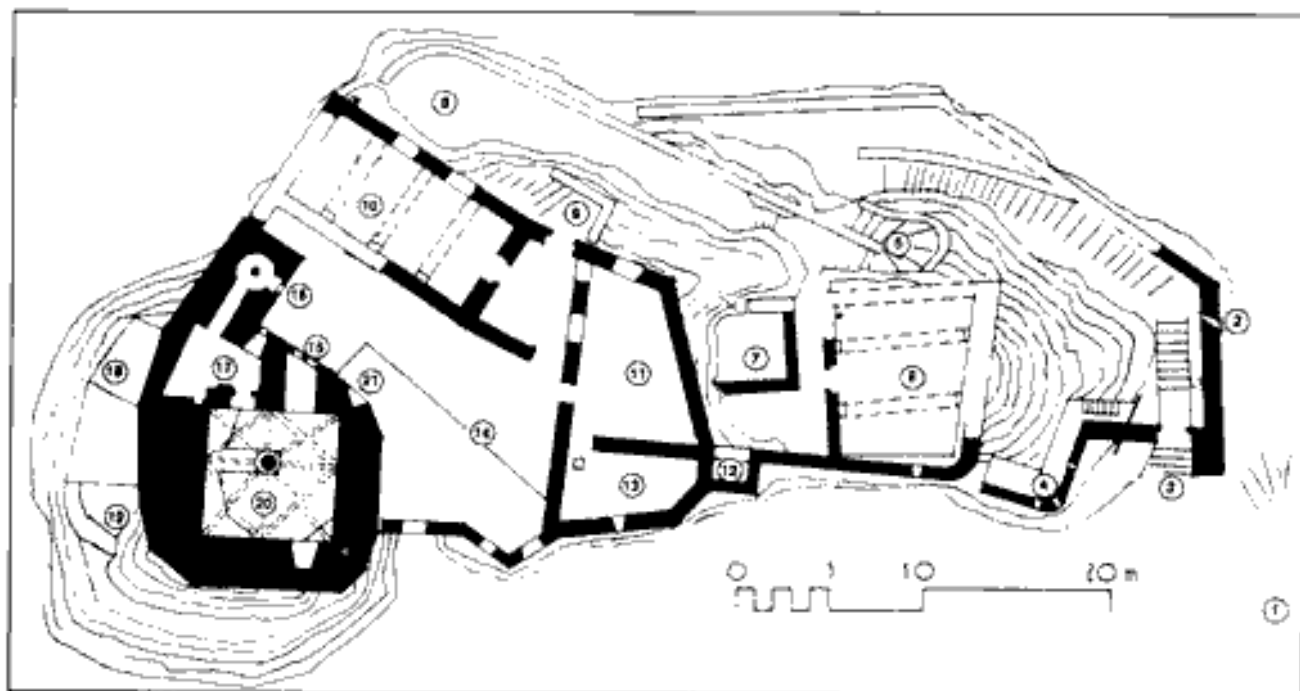
Queribus, plán hradu
